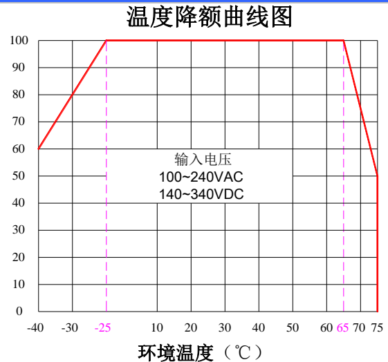
工作环境温度降额曲线图
