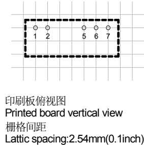
建议印刷板图
