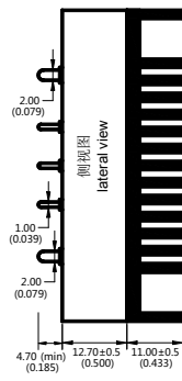
50-75W 散热片 (1)
