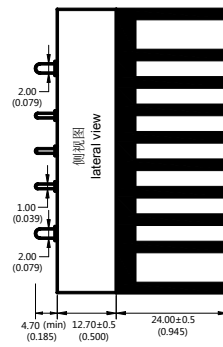
100-150W 散热片 (2)
