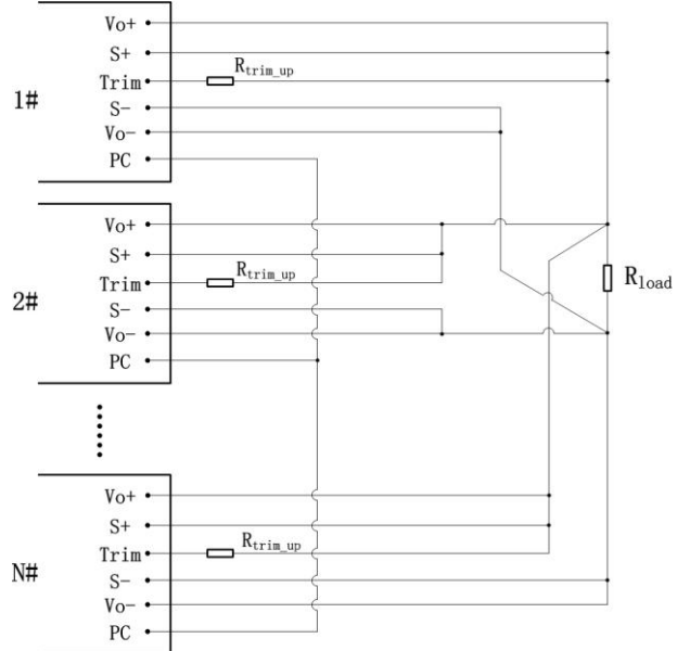
图16: 多模块并联使用配置
