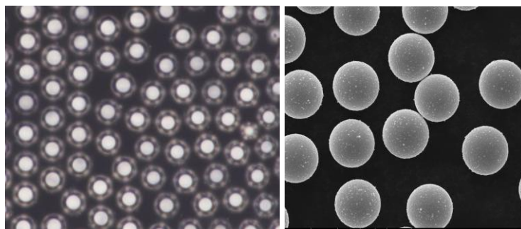
FaraBead® 导电镍球光学显微镜和 SEM 电镜图
