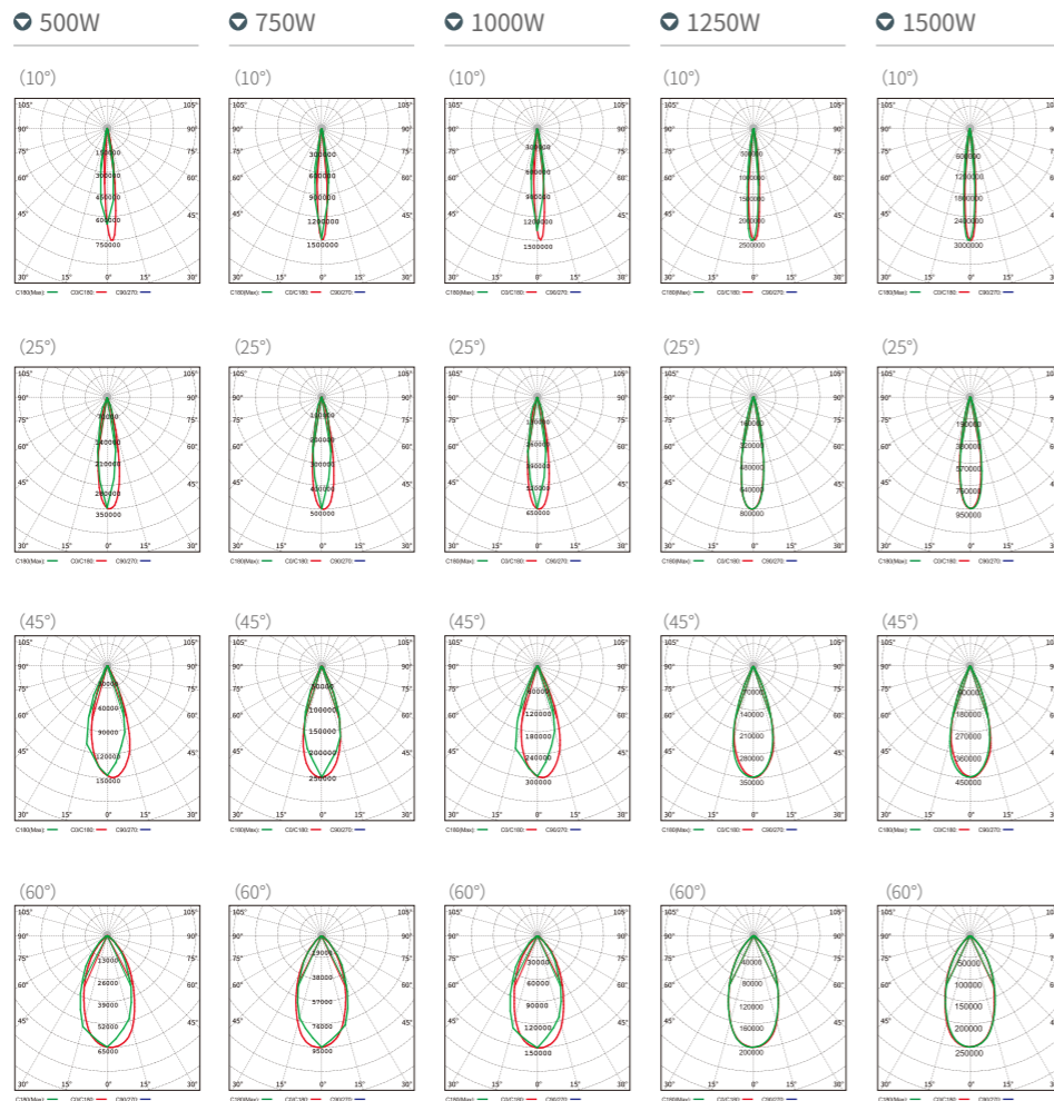
配光曲线图 (单位:cd)
