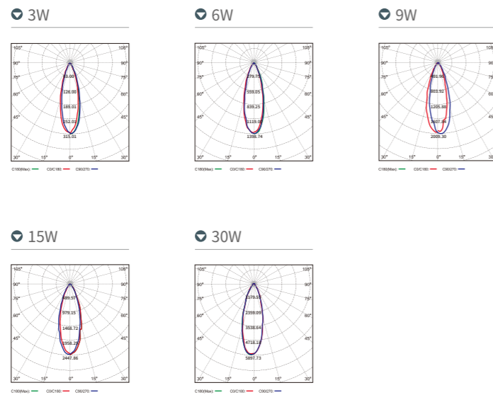
配光曲线图 (单位: cd)
