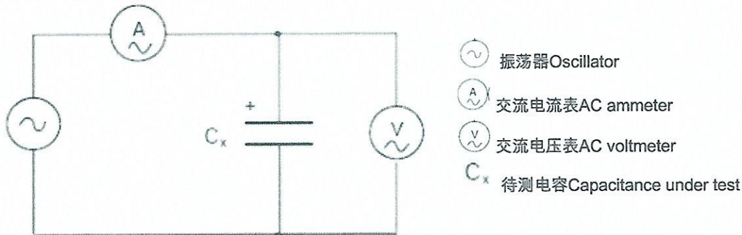
图3- 交流阻抗方法电路 AC impedance method circuit
