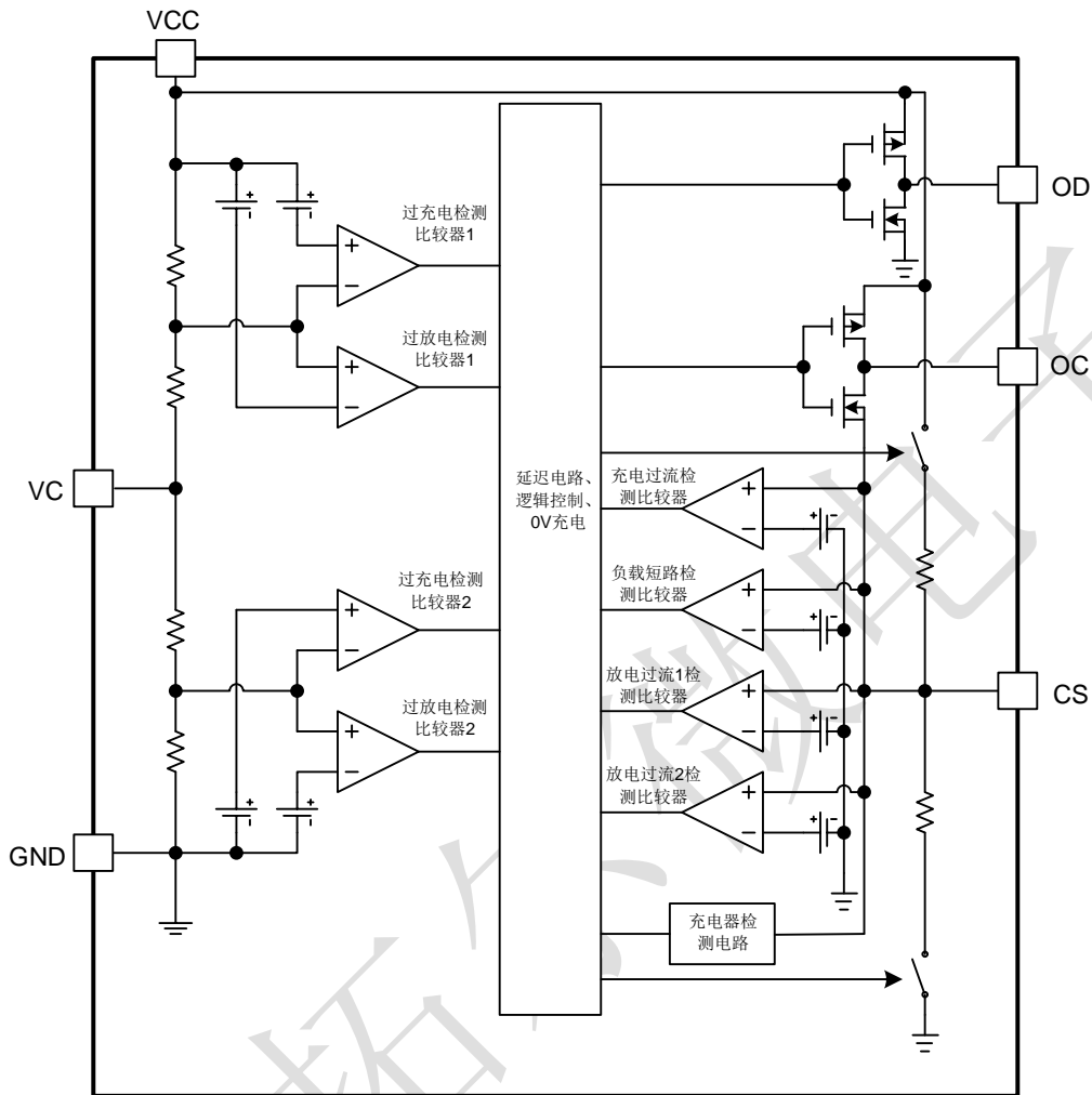
图 2 SIT8252 功能框图
