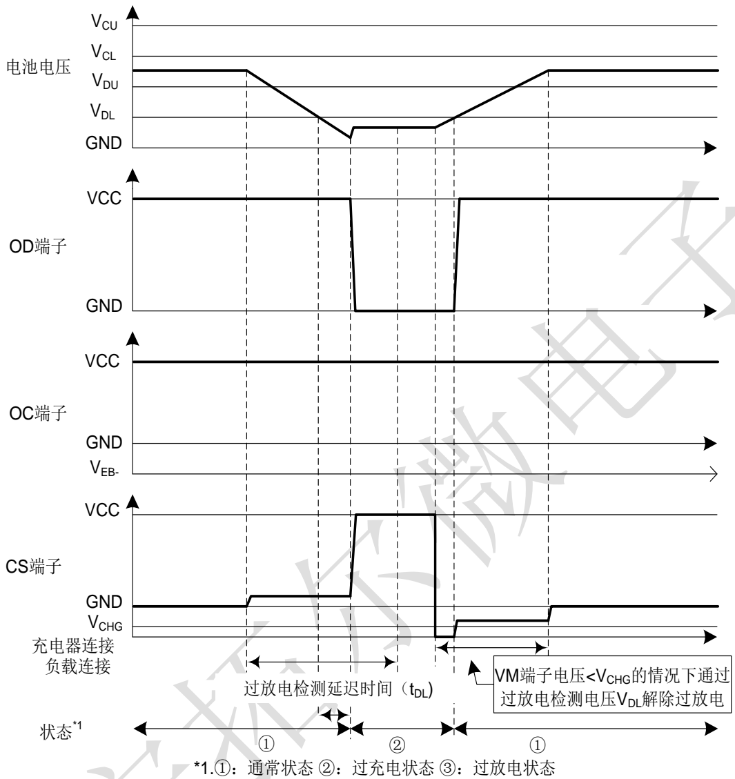
图 5 充电器检测
