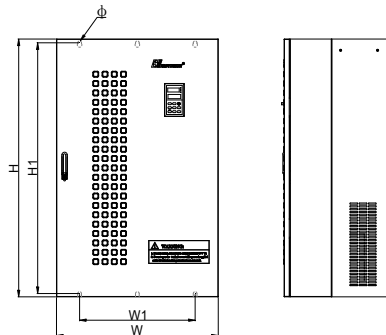
(c): 11KW~75KW 规格尺寸
