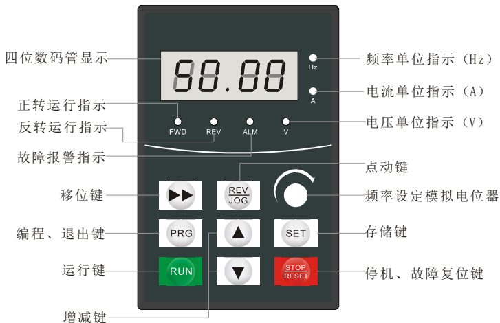
图 4-3 RKB 操作键盘示意图
