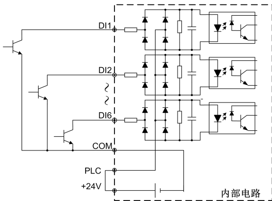
图 3-27 内部电源供电 NPN 图 (0C)
