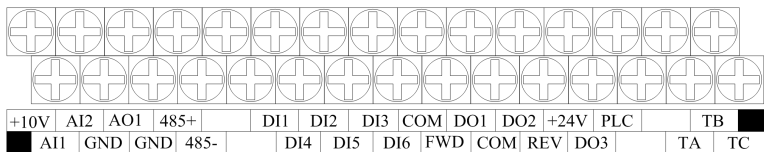
图 3-20 控制板端子排列顺序图(11KW 以上控制板)
