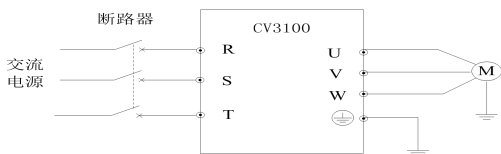
图 3-11 主回路简单配线
