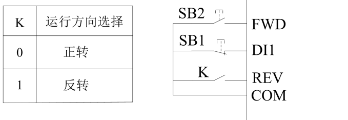
图 6-14 三线式控制模式 2
