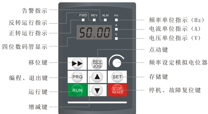
图 4-2 LKD 操作键盘示意图
