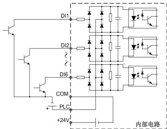
图 3-28 外部电源供电 NPN 图 (0C)
