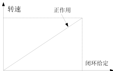
图 6-22 正特性示意图
