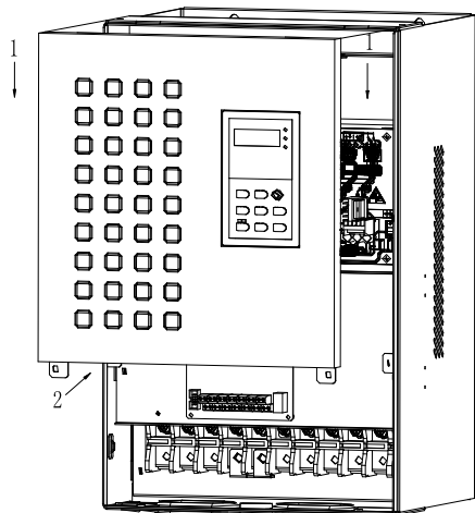
图 3-10 盖板的安装
