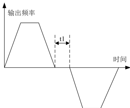
图 6-8 正反转死区时间
