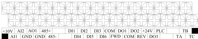
图 3-19 控制板端子排列顺序图(0.7~7.5KW 控制板)
