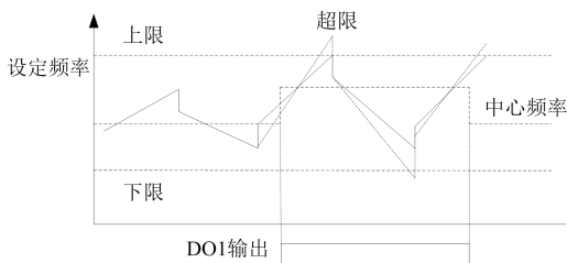
图 6-15 摆频运行上下限限制示意图
