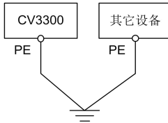
图3-13 接地示意图2
