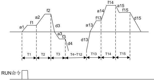
图6-46 PLC单循环后停机方式
