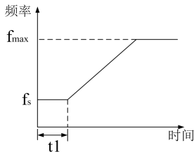
图6-8 起动机频率与起动机时间示意图
