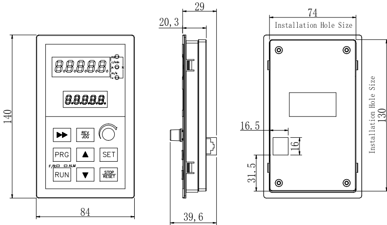
图 2-1 CV3300-RKD 键盘尺寸规格
