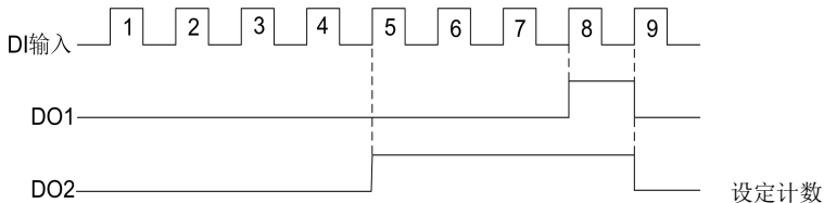
值给定和指定计数值给定示意图
