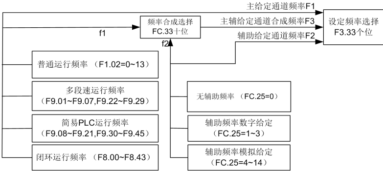
图6-65 给定频率合成示意图
