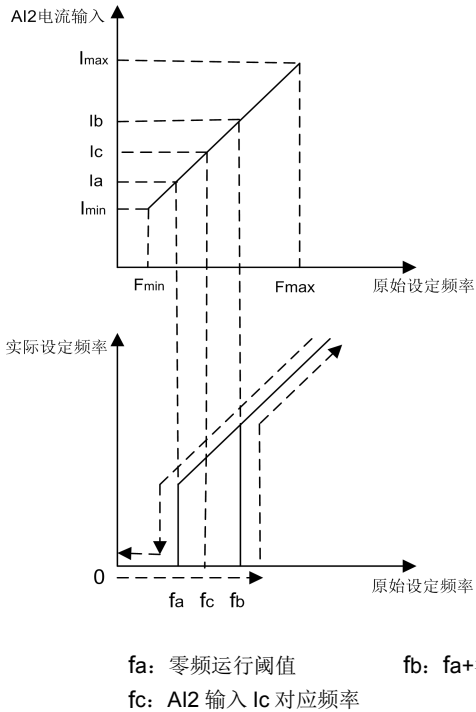
图6-61 零频回差运行
