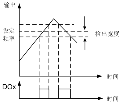
图6-30 频率到达信号输出示意图
