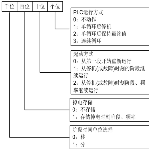
图6-45 简易PLC运行方式选择
