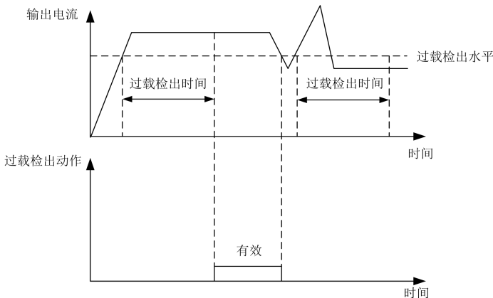
图6-54 过载预警检出功能示意图
