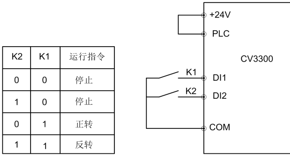
图6-26 两线式运转模式2
