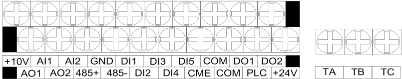
图 3-4 CV3300-4T0055G/4T0075P 及以上控制板端子排列顺序图
