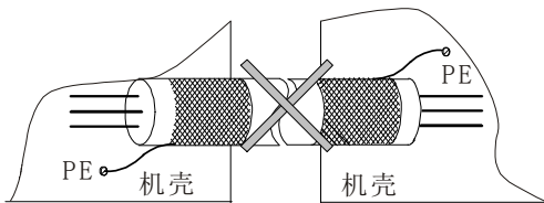
图3-17 错误的屏蔽接地方法
