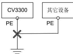
图3-15 接地示意图4
