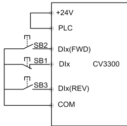
图6-27 三线式运转模式1
