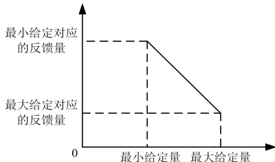
图6-41 给定、反馈曲线示意图2
