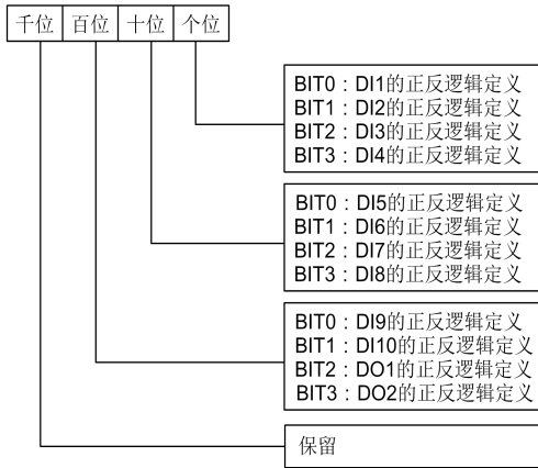
图6-32 端子正反逻辑设定
