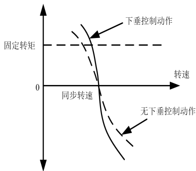
图6-60 下垂控制电机特性
