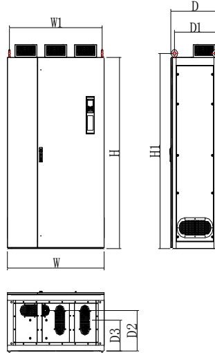
(f) F 规格尺寸
