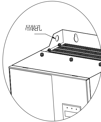
图 2-7 钣金结构吊装示意图 表 2-2 壁挂式安装支架选配表
