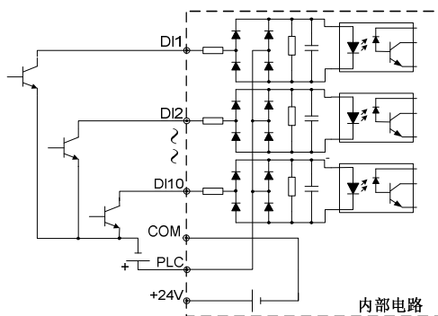
图 2-24 内部电源供电 NPN 图 (OC)
