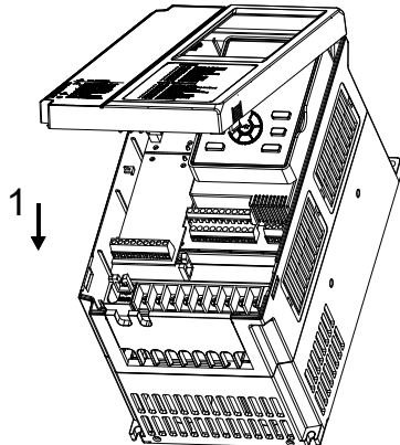
图 2-11 盖板的安装
