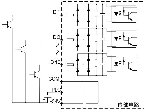
图 2-27 外部电源供电 PNP 图 (OE)
