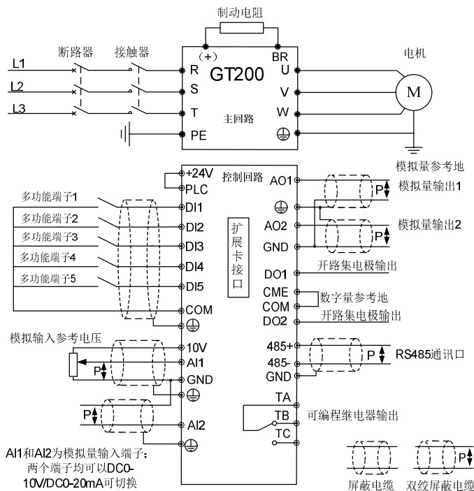
图 2-22 基本运行配线图
