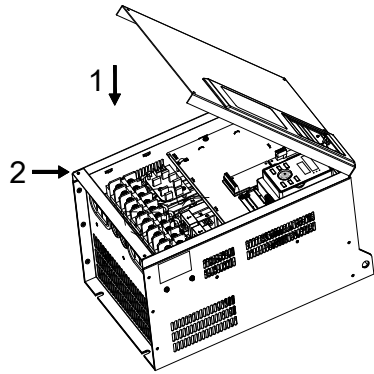
图 2-13 盖板的安装
