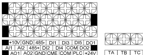
图 2-19 GT200-4T0040G/4T0055P 及以下控制板端子排列顺序图
