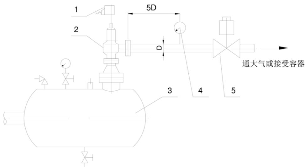
图5 具有附加背压时的推荐试验布置
