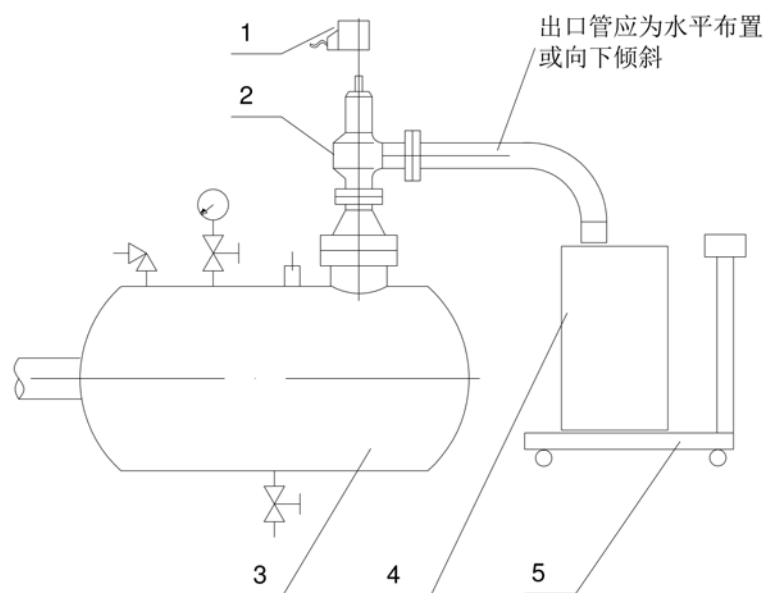
图3 称量冷凝液方法，背压为大气时的推荐试验布置
