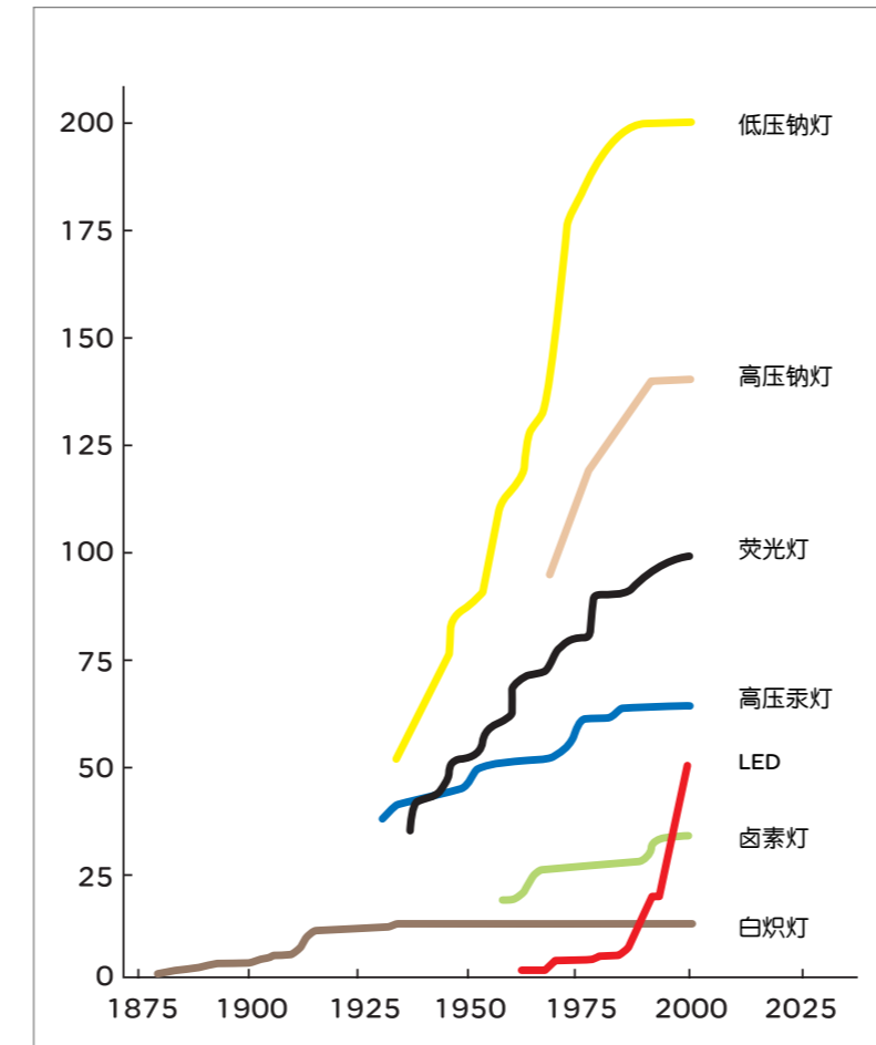
各种光源发光效率的发展历史进程
