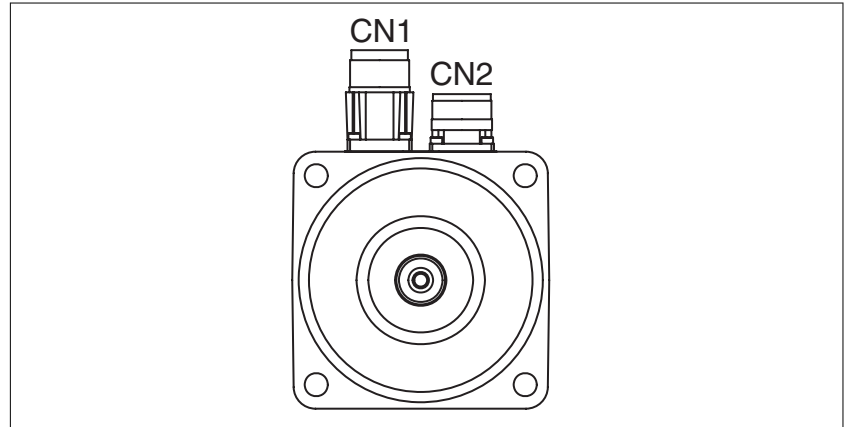
图 12: 连接概况
