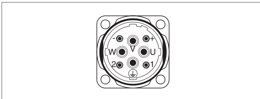
图 14: 电机接头 M40 引脚分配
