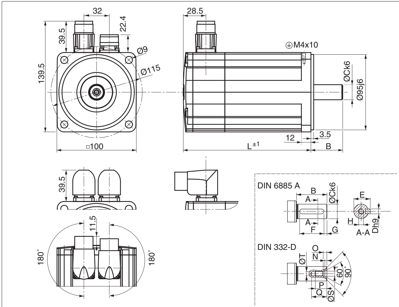
图 3: BMH100 尺寸
