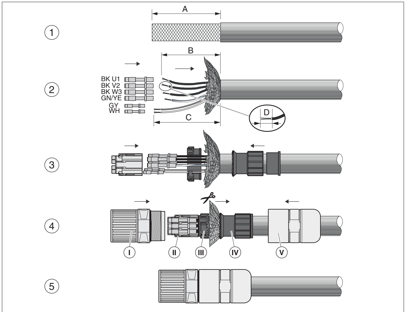
图 17: 用电机插头 M23 给电机电缆装配
