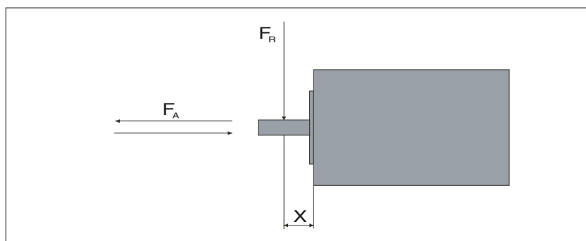
图 7: 轴负载
