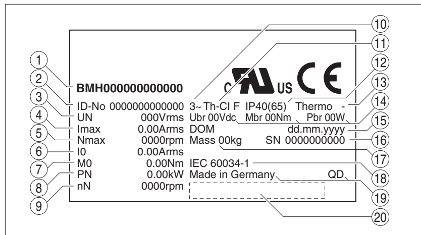
图 1: 铭牌
