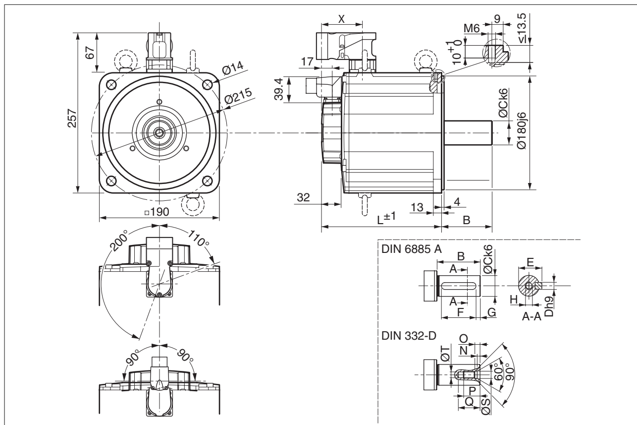
图 5: BMH190 尺寸
