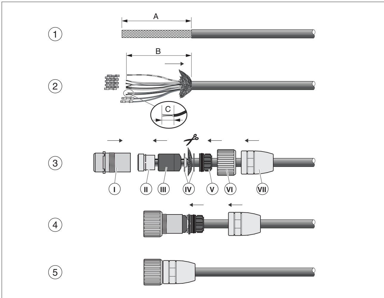
图 16: 请用 M23 编码器插头连接编码器电缆
