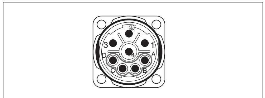
图 13: 电机接头 M23 针脚分配
