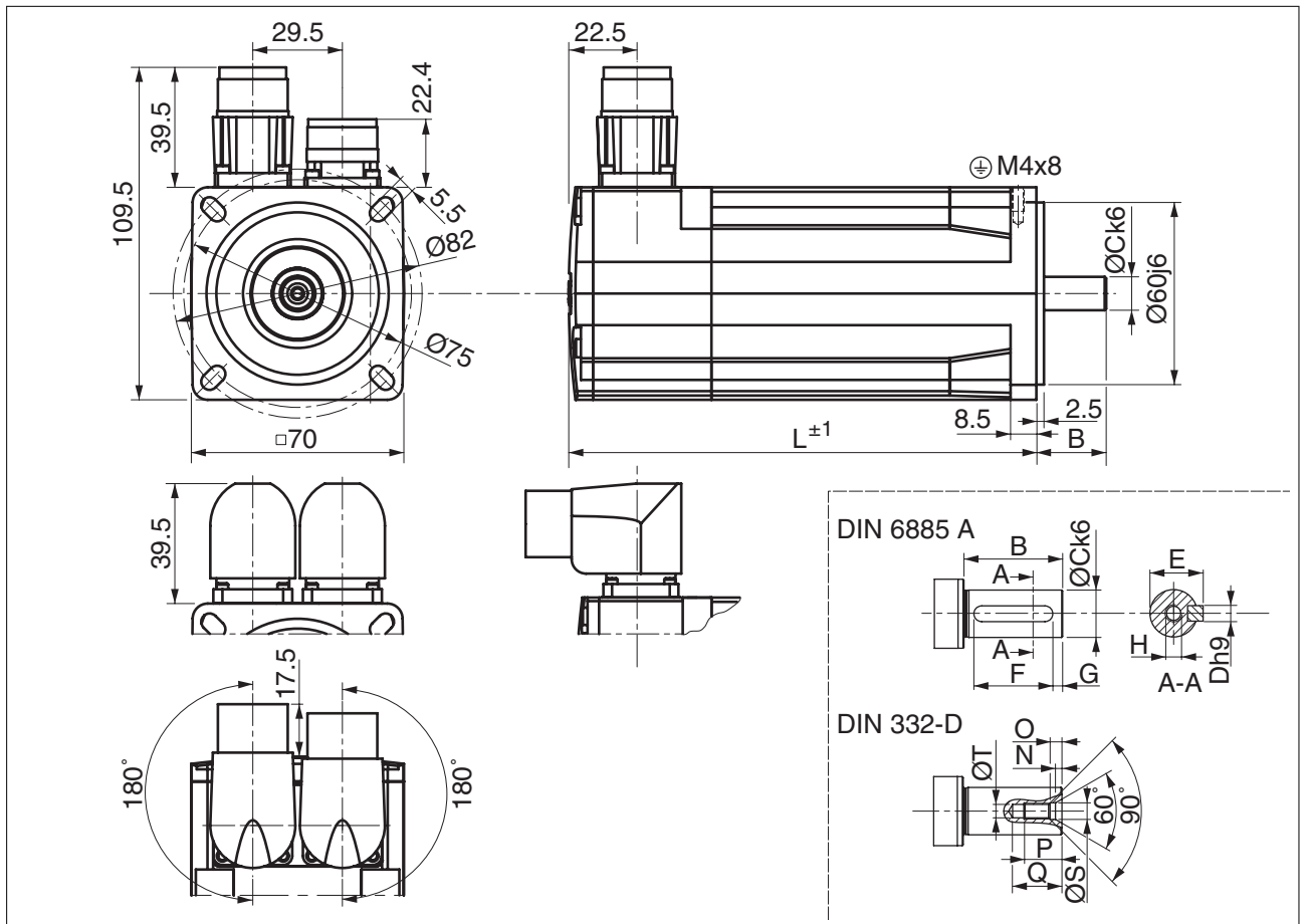
图 2: BMH070 尺寸
