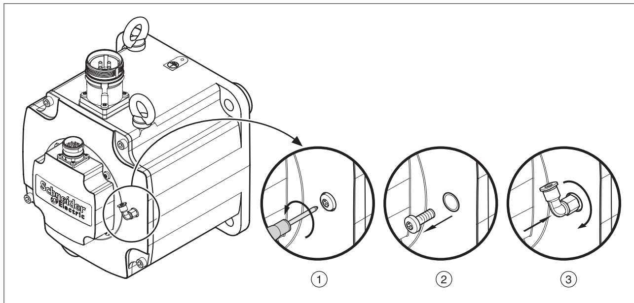
图 11: L 插头连接 BMH190 的安装
