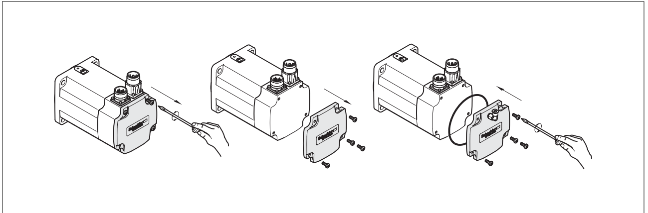
图 10: 安装 IP67 套件
