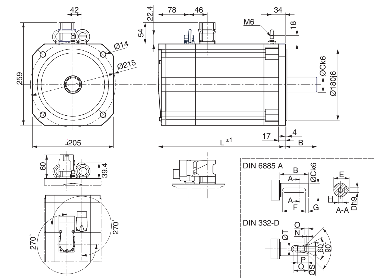
图 6: BMH205 尺寸
