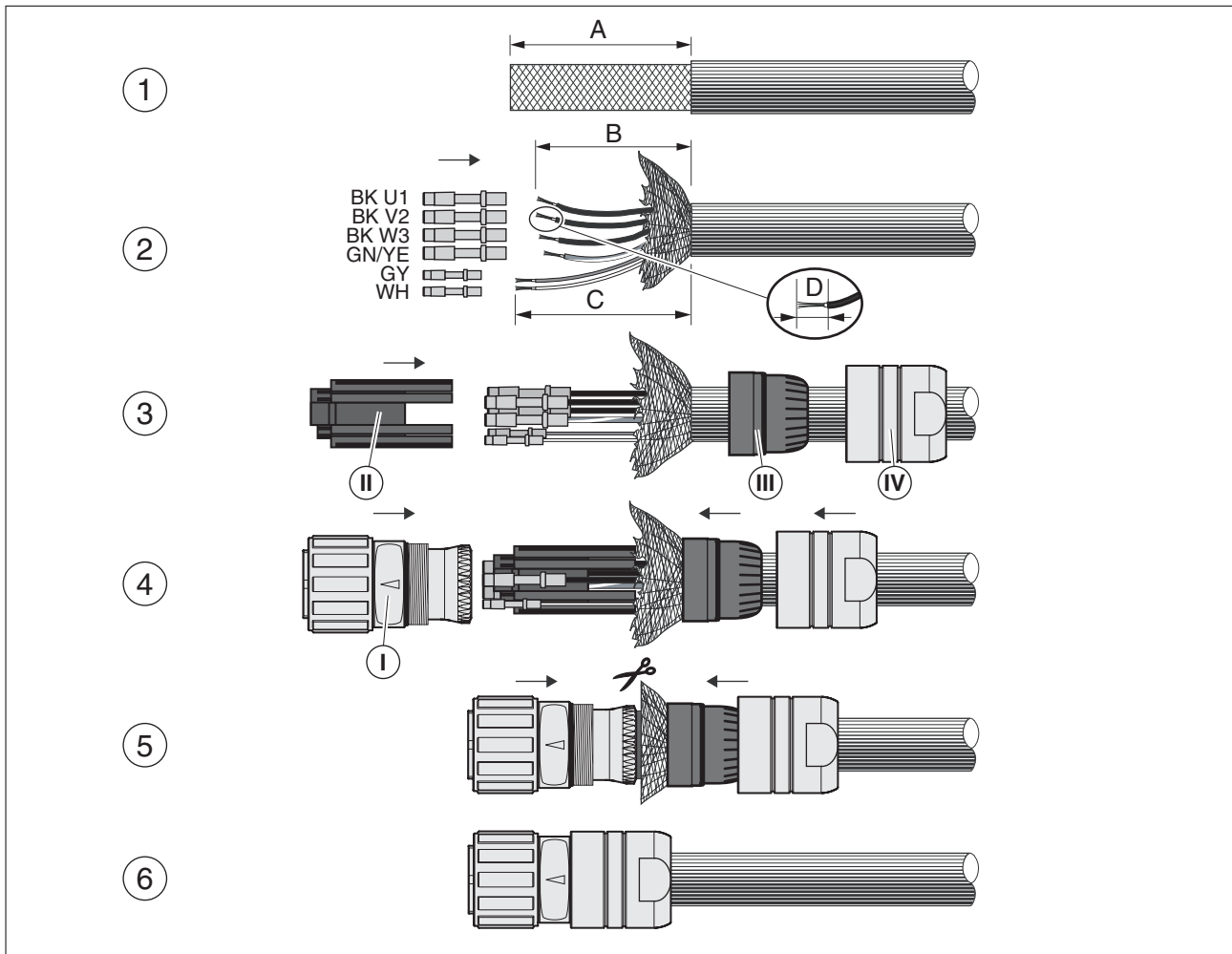
图 18: 用电机插头 M40 给电机电缆装配
