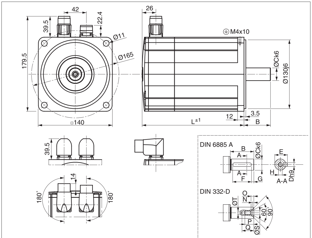
图 4: BMH140 尺寸
