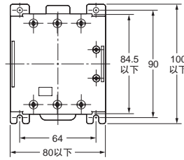
注: 有端子盖安装状态
