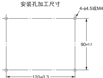
安装孔加工尺寸
