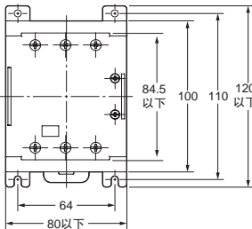
注: 有端子盖安装状态
