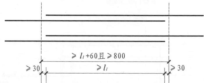
板后浇带HJD贯通钢筋构造
