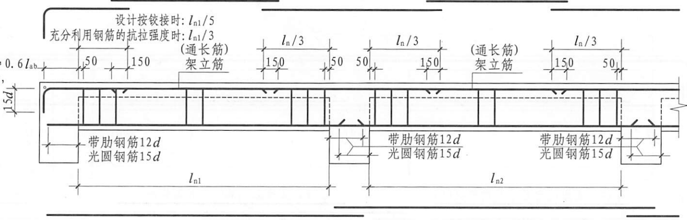
非框架梁配筋构造 (梁上部通长筋连接要求见注2)
