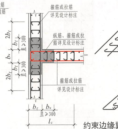
剪力墙水平分布钢筋计入约束边缘构件 体积配箍率的构造做法
