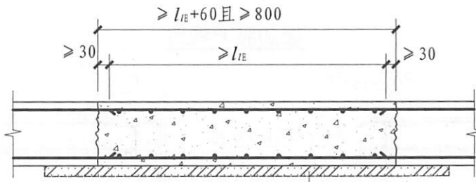
墙后浇带HJD贯通钢筋构造
