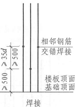
剪力墙边缘构件纵向钢筋连接构造
