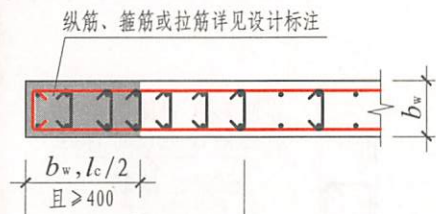
约束边缘暗柱 (二)
