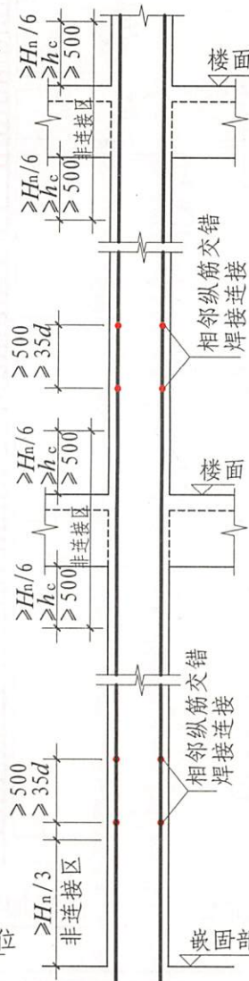
焊接连接
