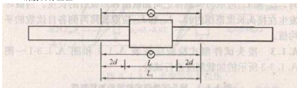
图 A.1.1 接头试件变形测量标距和仪表布置
