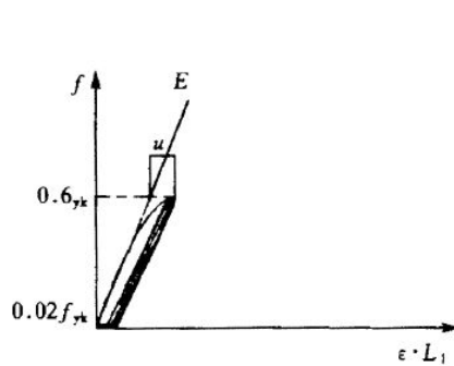
图 A.0.1-1 单向拉伸
