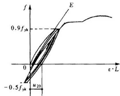
图 A.0.1-2 高应力反复拉压
