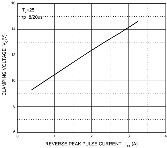
V_c ---- I_{PP}
