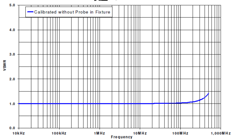
典型 VSWR
