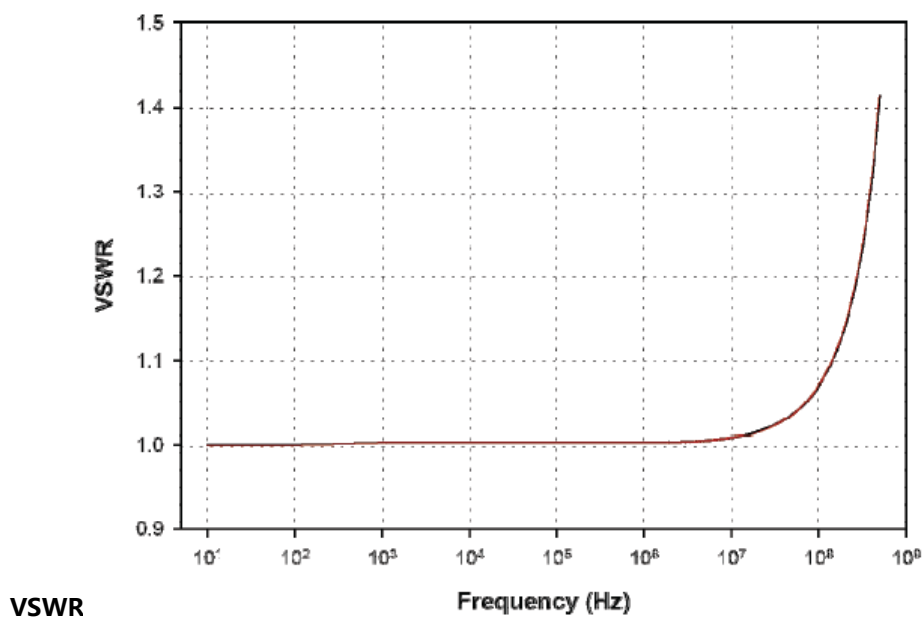
典型 VSWR
