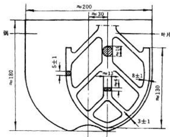
图 1 搅拌机
