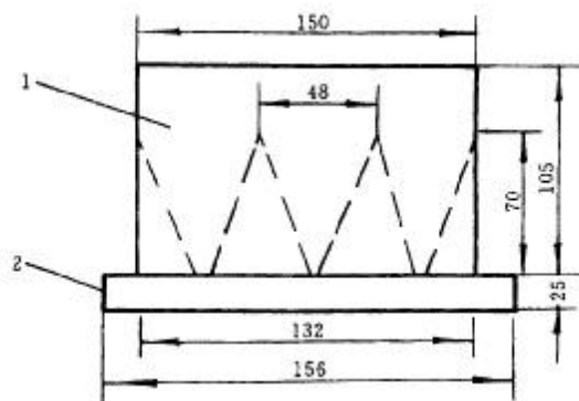
1- 漏斗;2- 模套
