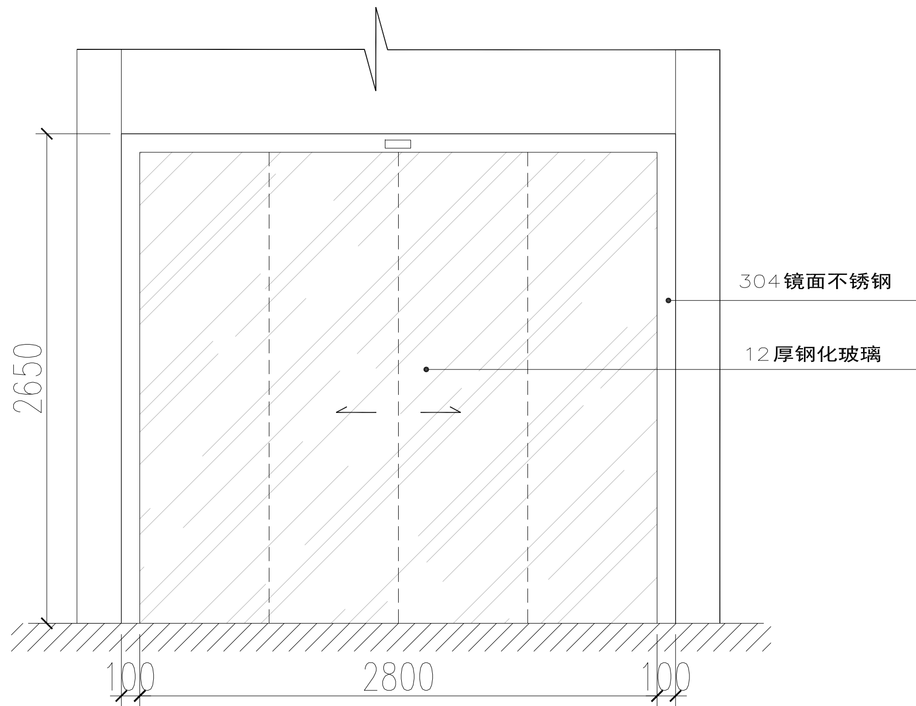
小卖部西侧玻璃感应门示意图
