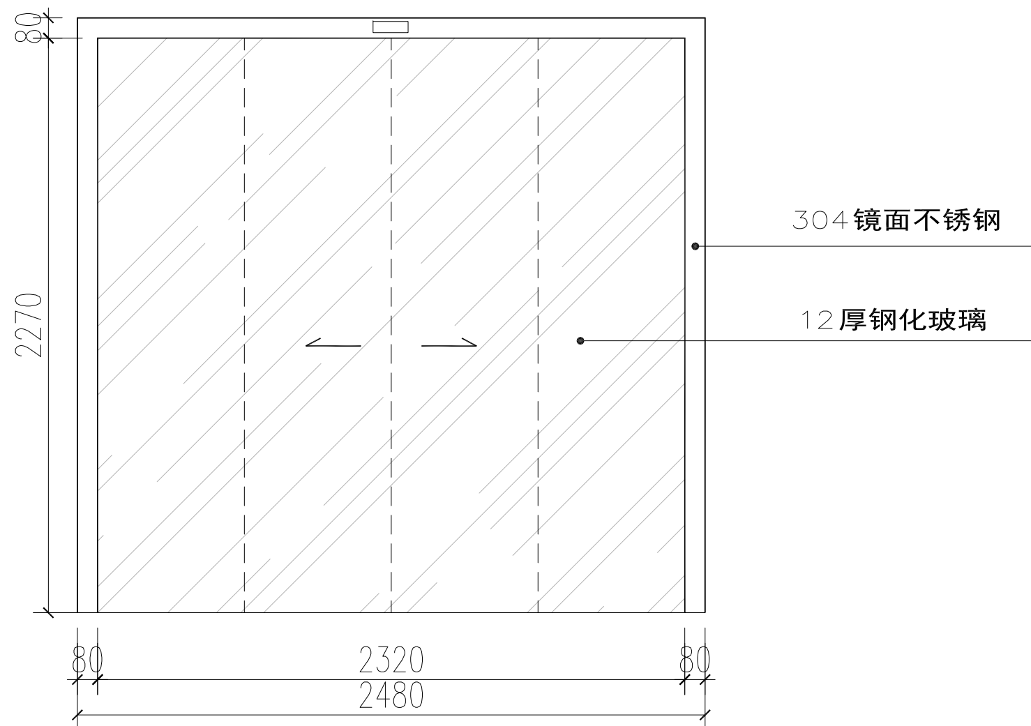
大厅（下坡踏步处）感应门示意图
