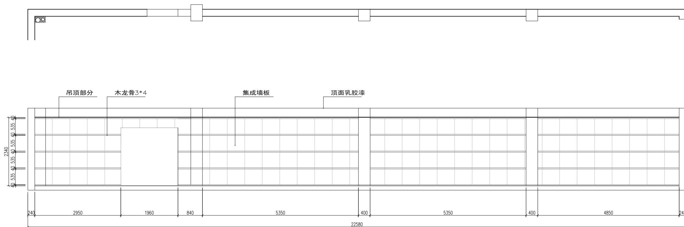
PLAN 休息区南立面图
