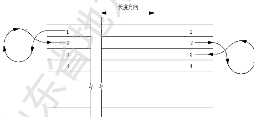
图2 施工作业场地较窄时冲击碾压路线示意图
