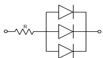
电路模式/Circuit model B
