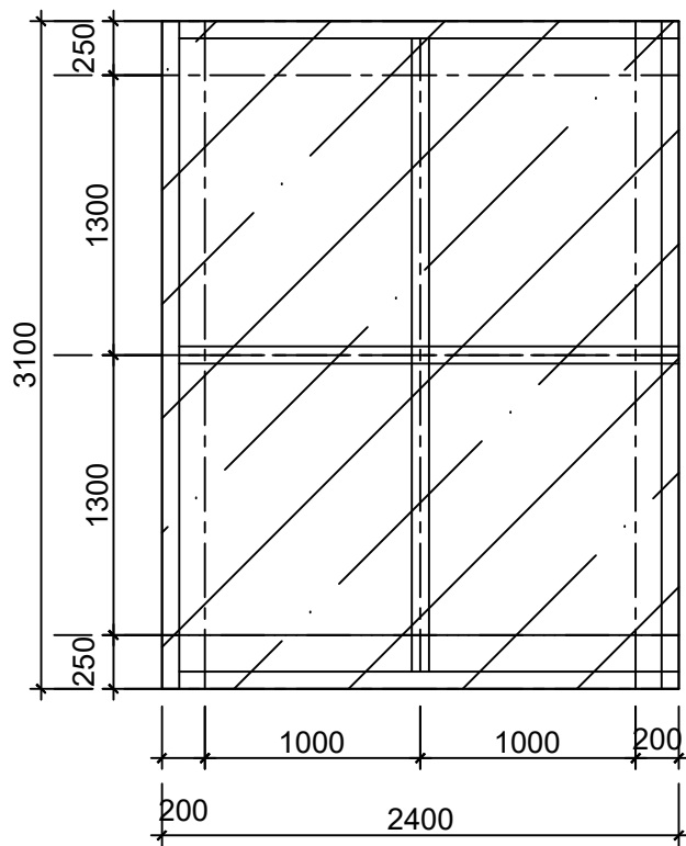
雨棚骨架平面图
