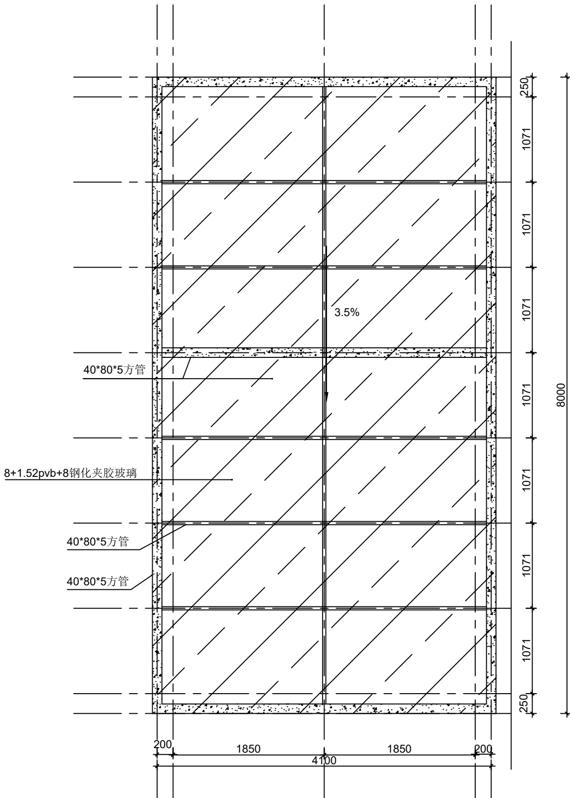
雨棚骨架平面图
