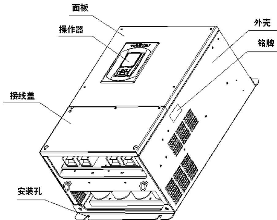
图 2-6 A4~A9 规格
