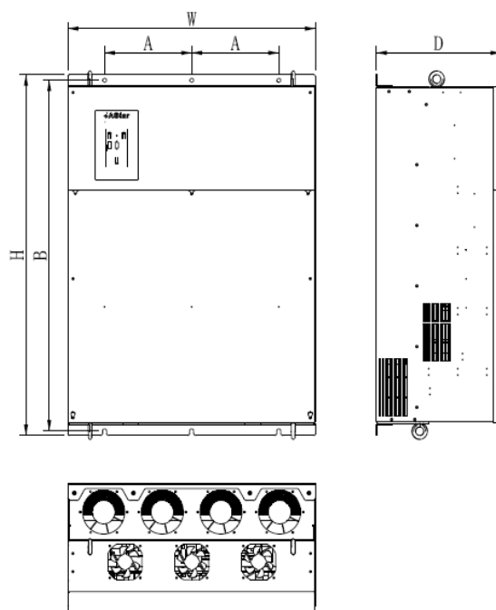
图 2-11 A10~A11 变频器安装尺寸
