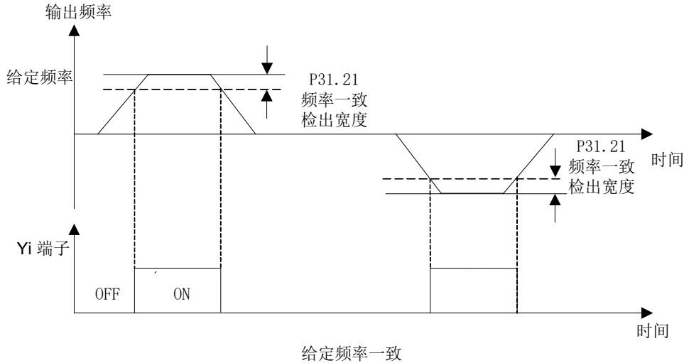
图 7-18 频率一致检出 1
