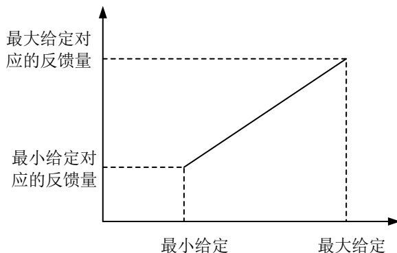
图 7-30 反馈正调节
