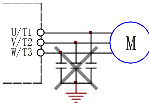
图 4-16 严禁在输出侧连接电容器的示意图
