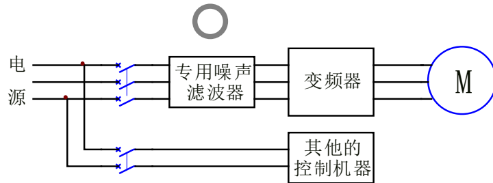
图 4-2 电源侧噪声滤波器的正确设置
