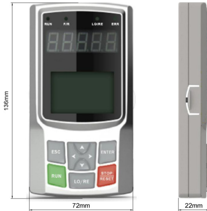
图 2-12 变频器的操作器尺寸
