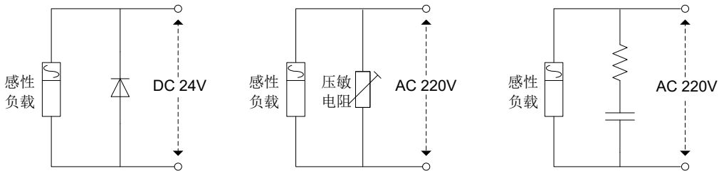
图 4-18 感性负载浪涌抑制器的应用
