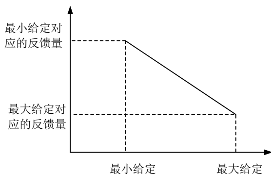
图 7-31 反馈负调节
