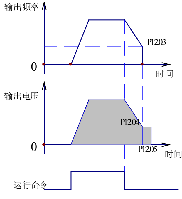
图 7-12 停车直流制动示意图
