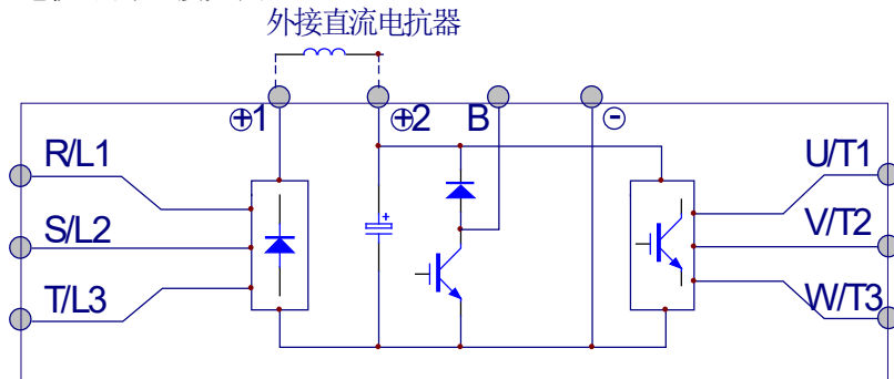
图 4-12 外接直流电抗器的连接图
