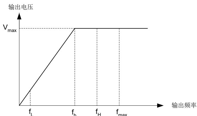
图 7-34 频率上下限示意图
