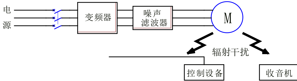
图 4-17 变频器输出侧噪声滤波器的接线
