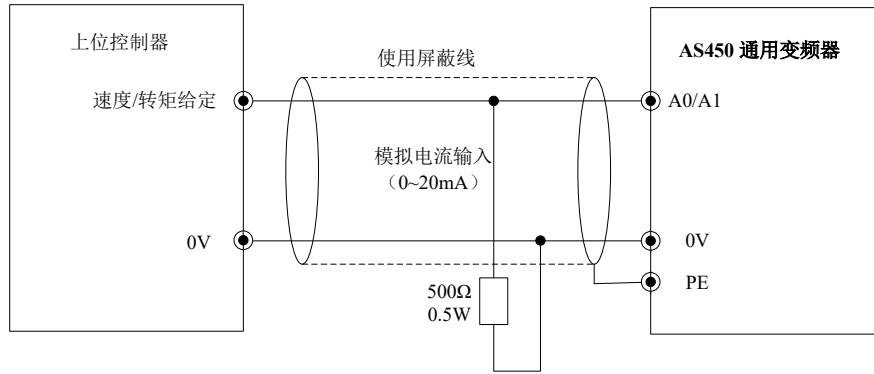
图 4-28 模拟量电流信号接线示意图
