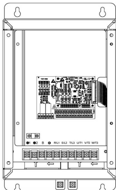
图 4-6 变频器内部视图
