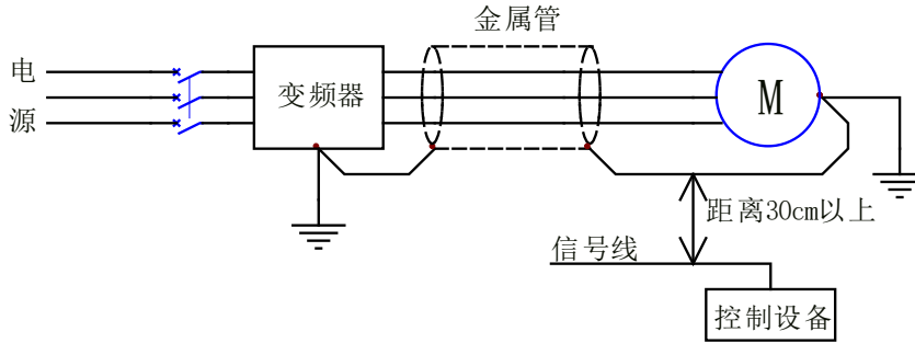
图 4-20 主回路配线的布置示意图 2
