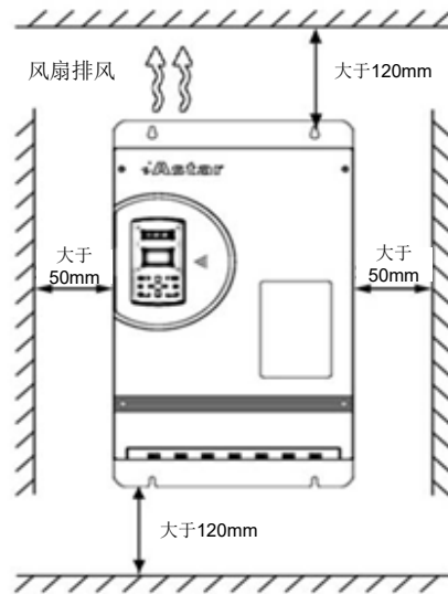
a) 37kW 及以下变频器的安装间距示意图
