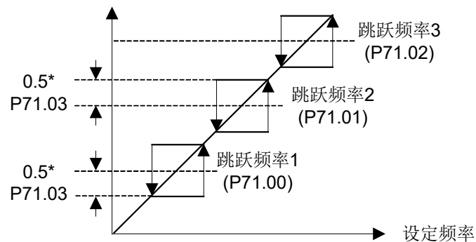
图 7-35 跳跃频率上下限
