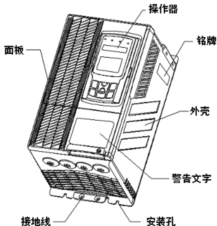
图 2-4 A1 规格
