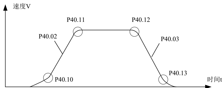
图 7-22 S 曲线在电机运行中的位置
