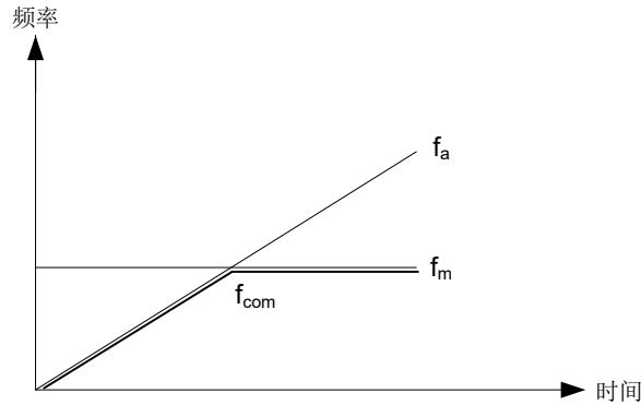
图 7-28 开环主辅给定运算 5
