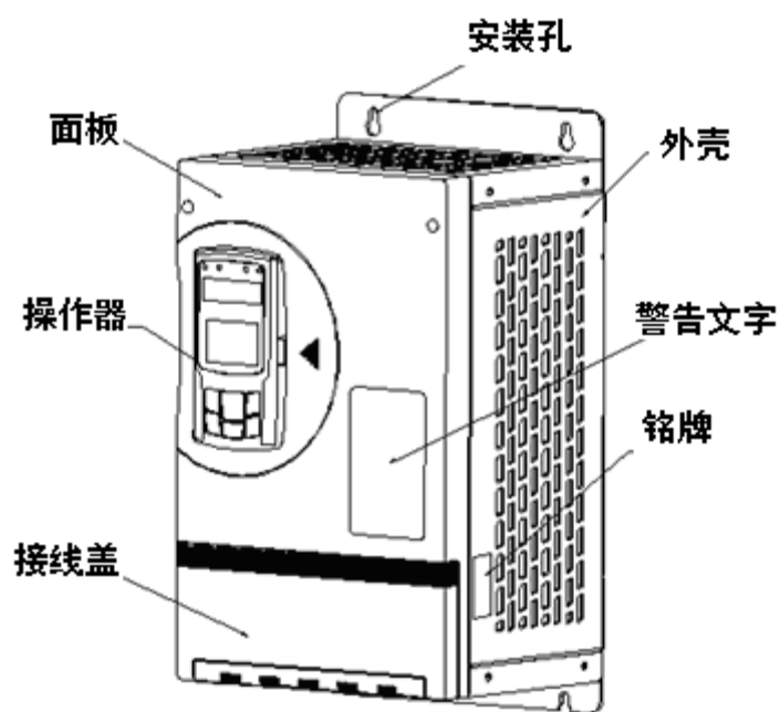
图 2-5 A2~A3 规格
