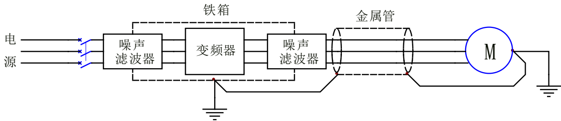
图 4-22 较完善的抗干扰措施
