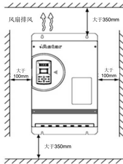
b) 45kW 及以上变频器的安装间距示意图
