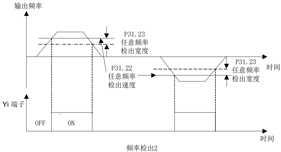
图 7-21 速度检出 2
