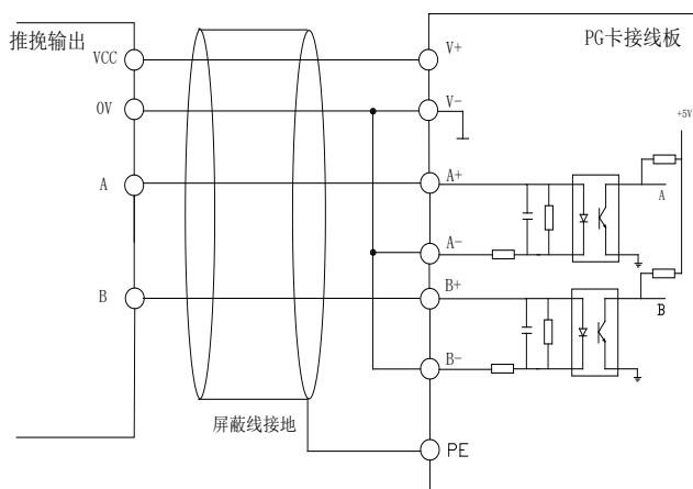
图 4-31 与编码器推挽信号的配线
