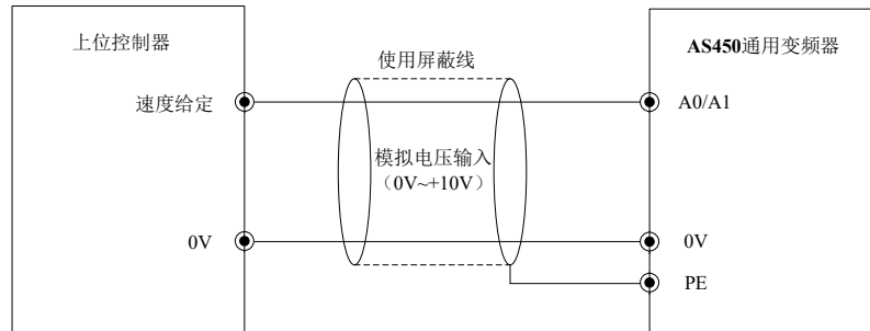
图 4-27 模拟量电压信号接线示意图
