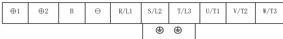
a) 22kW 及以下功率
