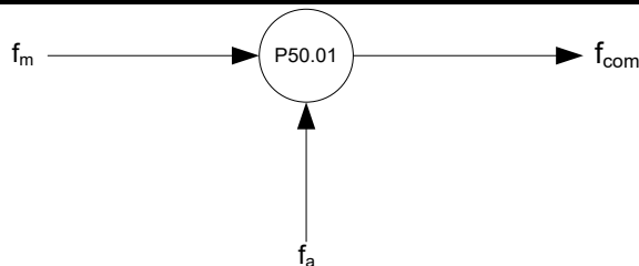
图 7-24 开环主辅给定合成示意图
