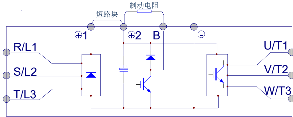
图 4-13 外接制动电阻的连接图
