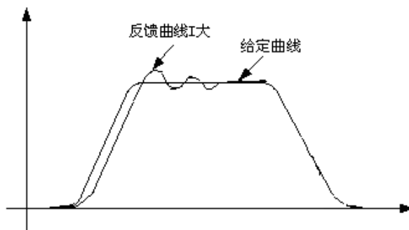
图 7-33 积分常数 I 对反馈跟踪的影响
