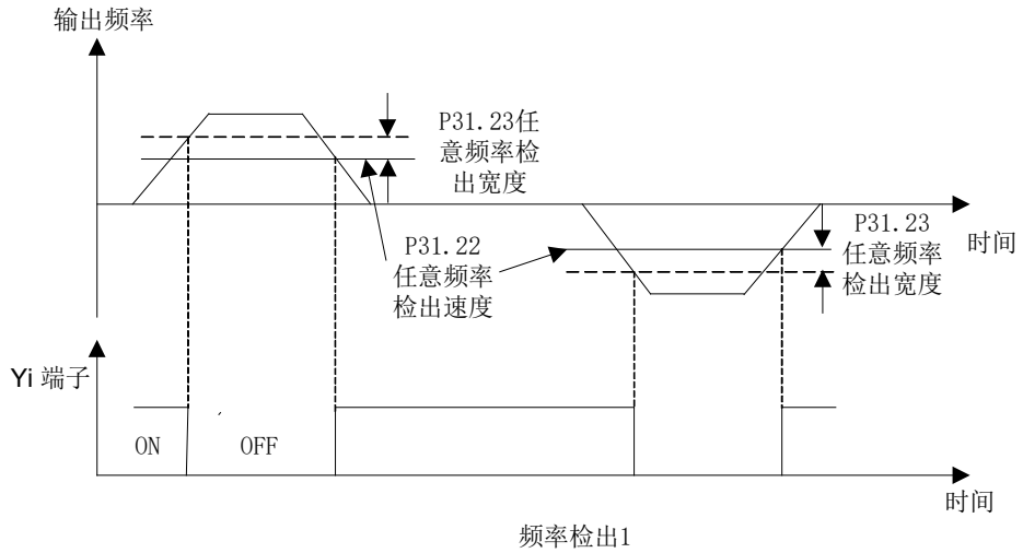
图 7-20 速度检出 1
