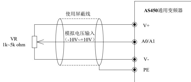
图 4-26 模拟量信号屏蔽线接线示意图
