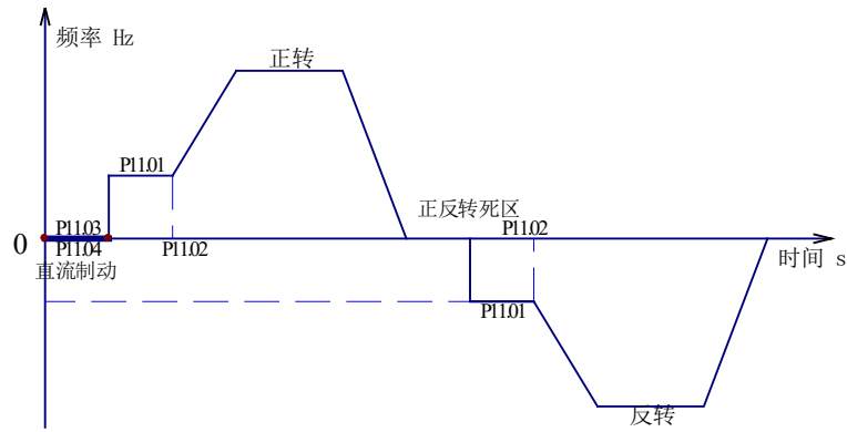
图 7-6 直流制动起动方式示意图
