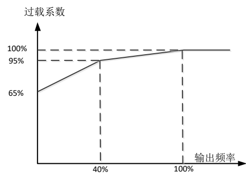
图 7-16 P23.00=2 时，过载降容系数
