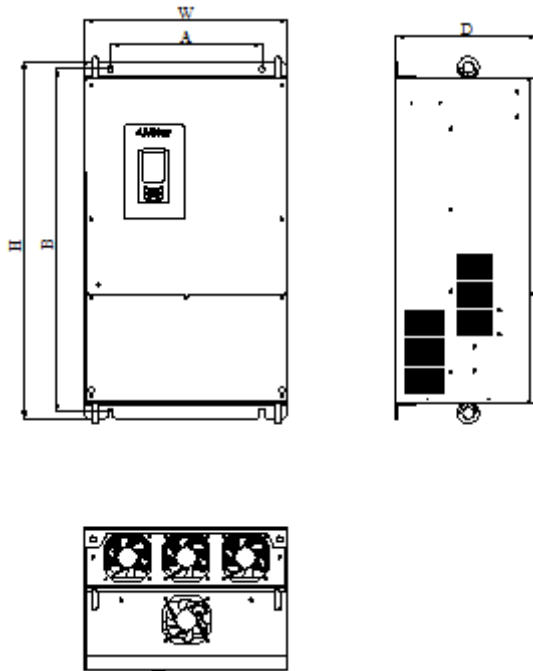
图 2-10 A4~A9 变频器安装尺寸
