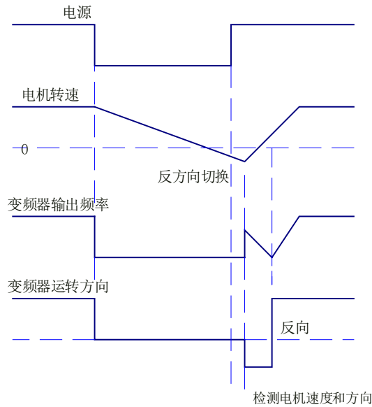
图 7-7 速度跟踪起动方式示意图
