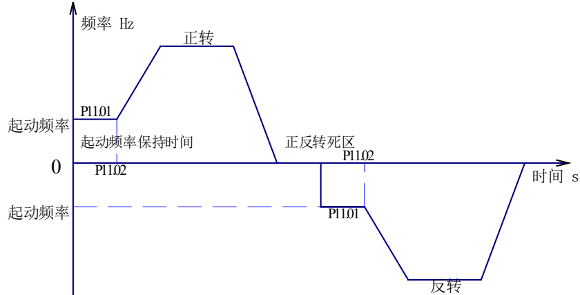
图 7-5 起动频率起动方式示意图
