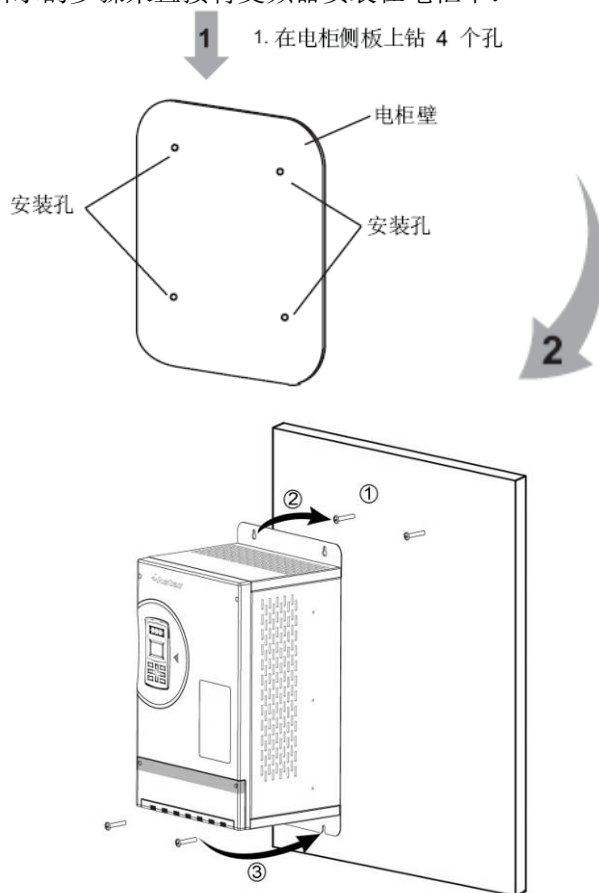
图 3-5 变频器的安装顺序图
