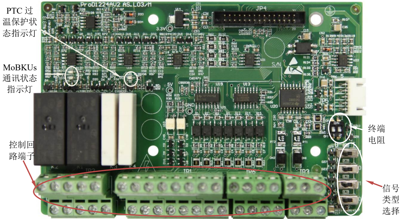
图 4-23 控制回路端子图片
