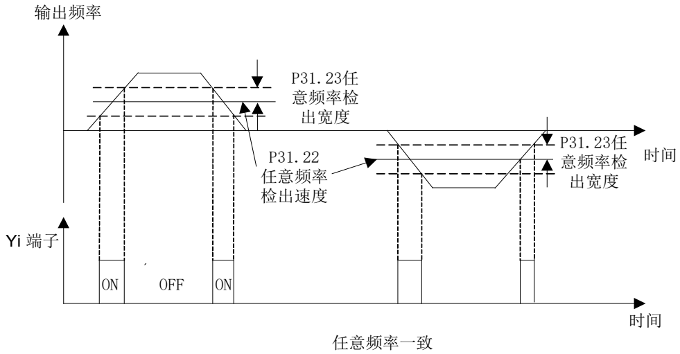
图 7-19 频率一致检出 2
