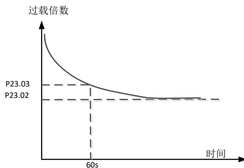
图 7-15 电机过热保护曲线图
