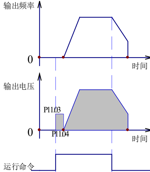
图 7-9 直流制动示意图
