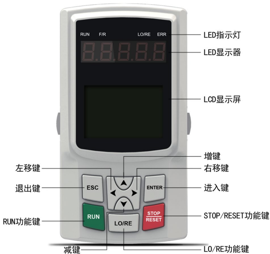
图 5-1 操作器各部分的名称和功能
