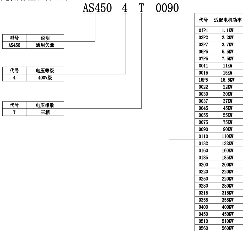
图 2-3 变频器型号说明
