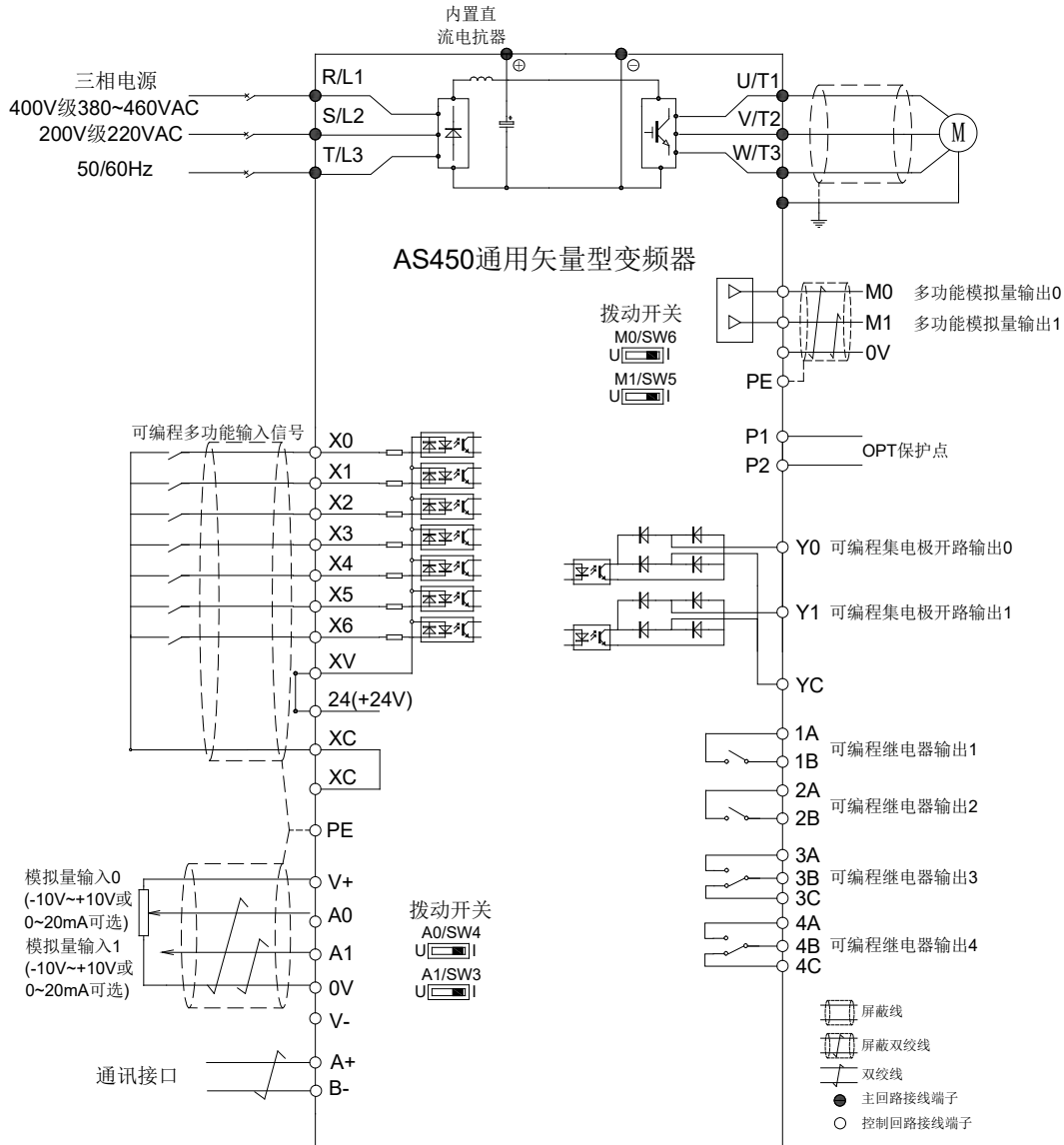
图 4-8 变频器端子配线示意图 2(22kW 以上)
