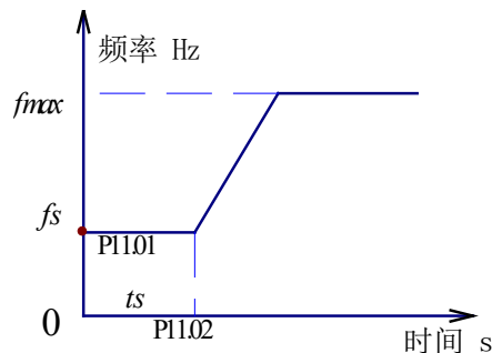
图 7-8 起动频率与起动时间示意图
