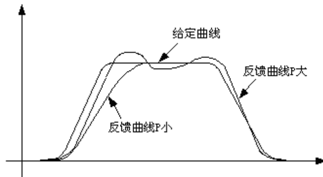
图 7-32 比例常数 P 对反馈跟踪的影响
