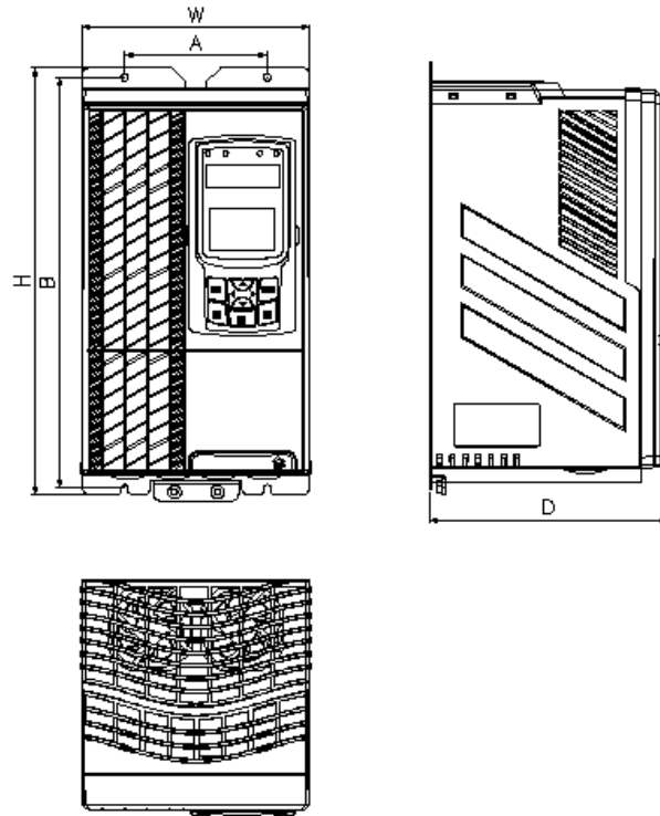
图 2-8 A1 规格变频器安装尺寸
