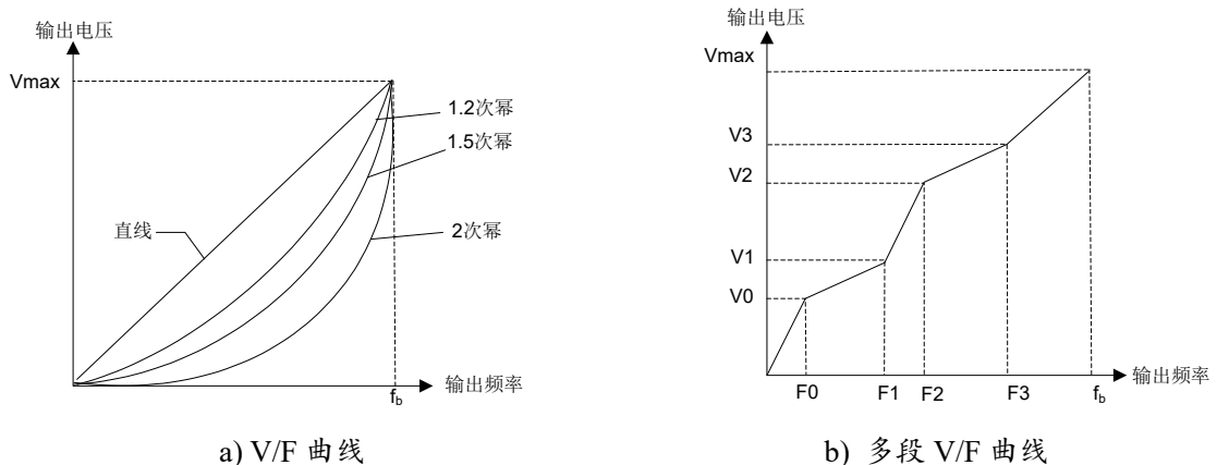
图 7-13 VF 曲线示意图
