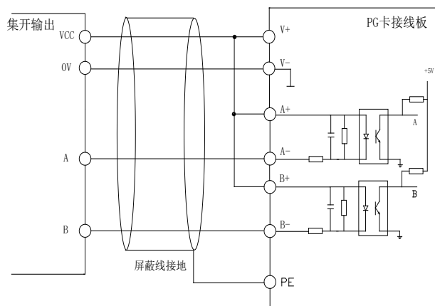
图 4-30 与编码器集电极开路信号的配线
