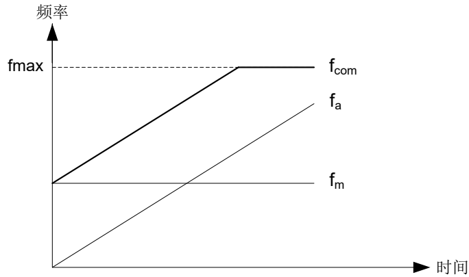
图 7-25 开环主辅给定运算 0
