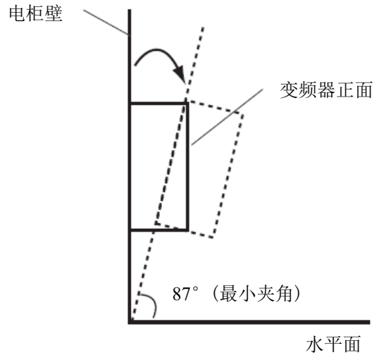
图 3-3 允许的安装夹角
