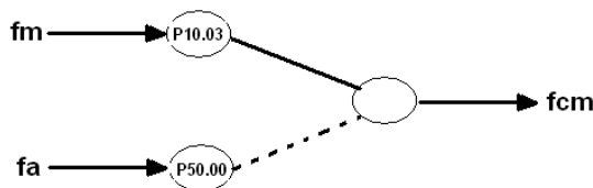
图 7-23 开环辅给定示意图
