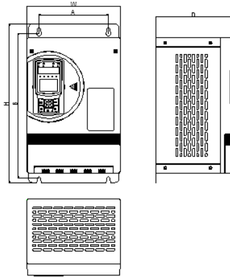
图 2-9 A2~A3 变频器安装尺寸
