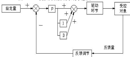
图 FA-1 模拟反馈控制系统示意图
