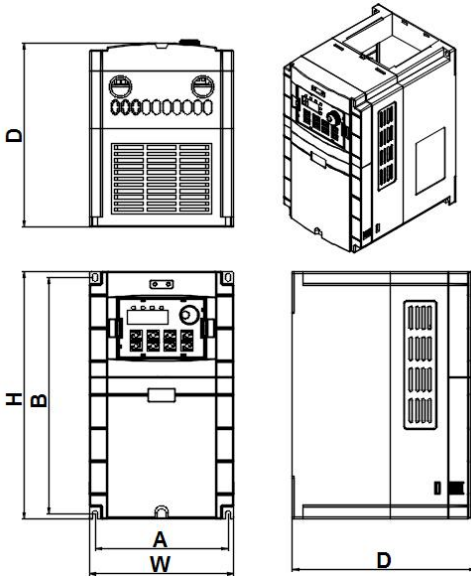
图 D-1 变频器 0.75KW~110KW 尺寸
