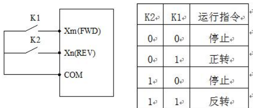
图 F4-2 二线式控制模式 1 示意图
