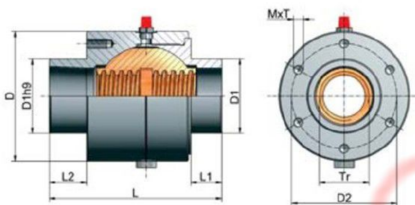
自对准螺母 SJA-.-PM
