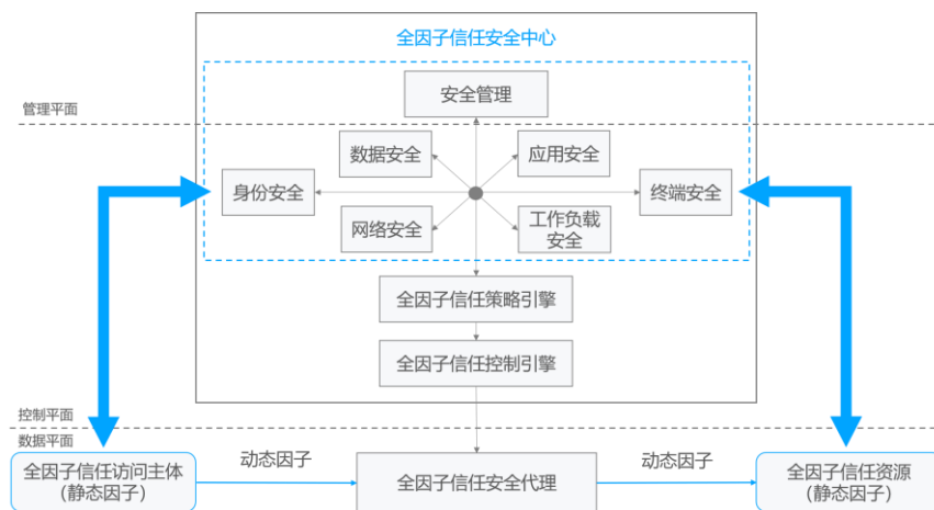
图 10 全因子信任安全架构
