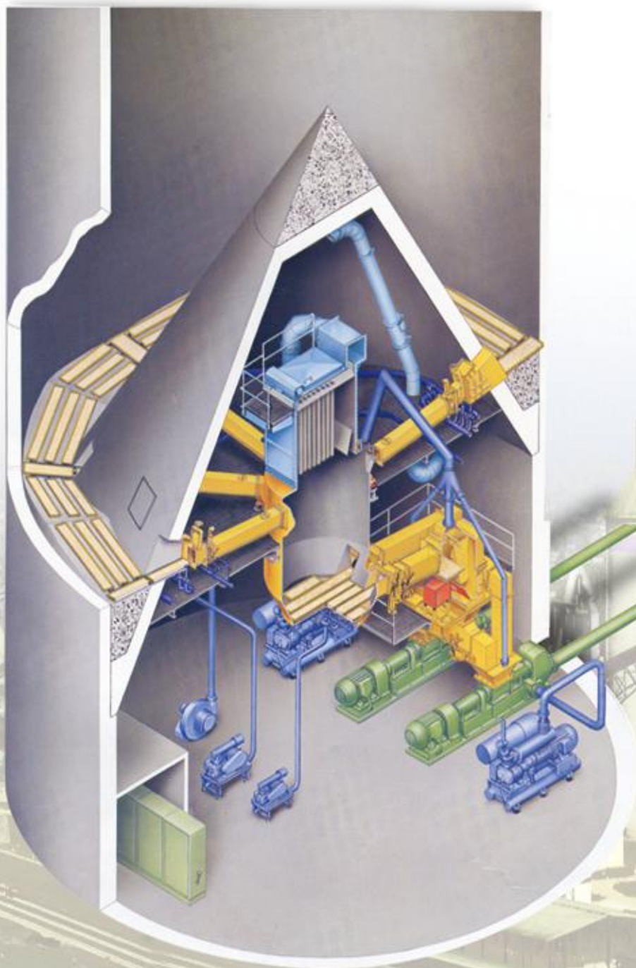
IBAU均化库
