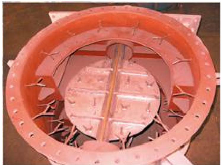
高温蝶阀
