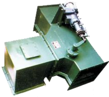
电动斜槽侧卸料阀
