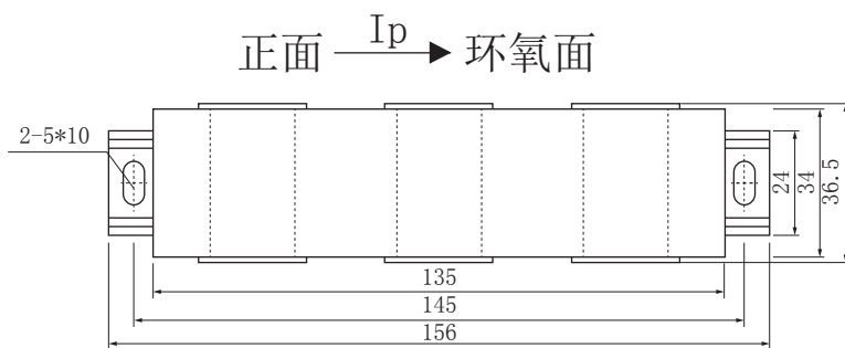
顶视图
