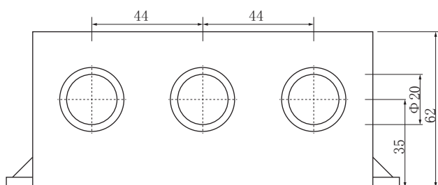
主视图
