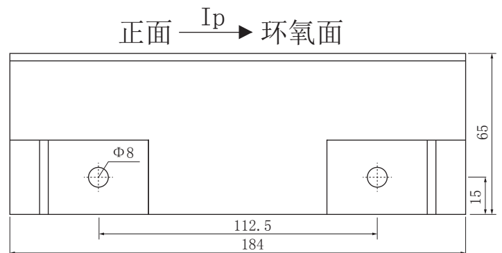
顶视图
