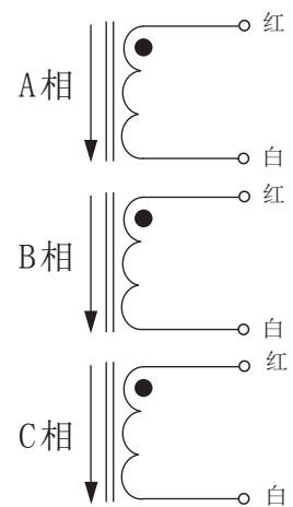
接线原理图：
