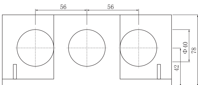
主视图
