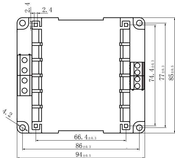
主视图
